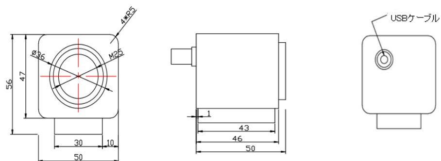
ACH200GS2-UVC 外形寸法
